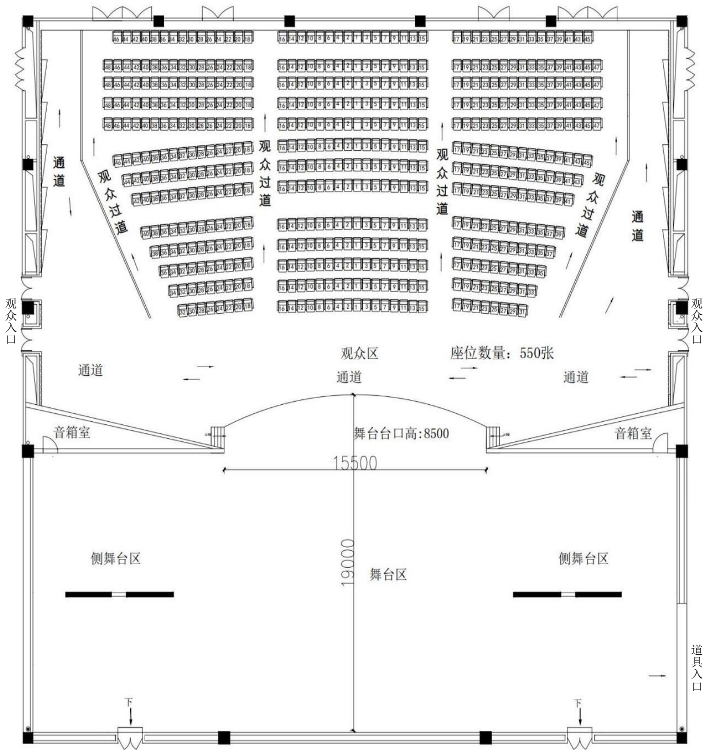
大剧场平面布置图
